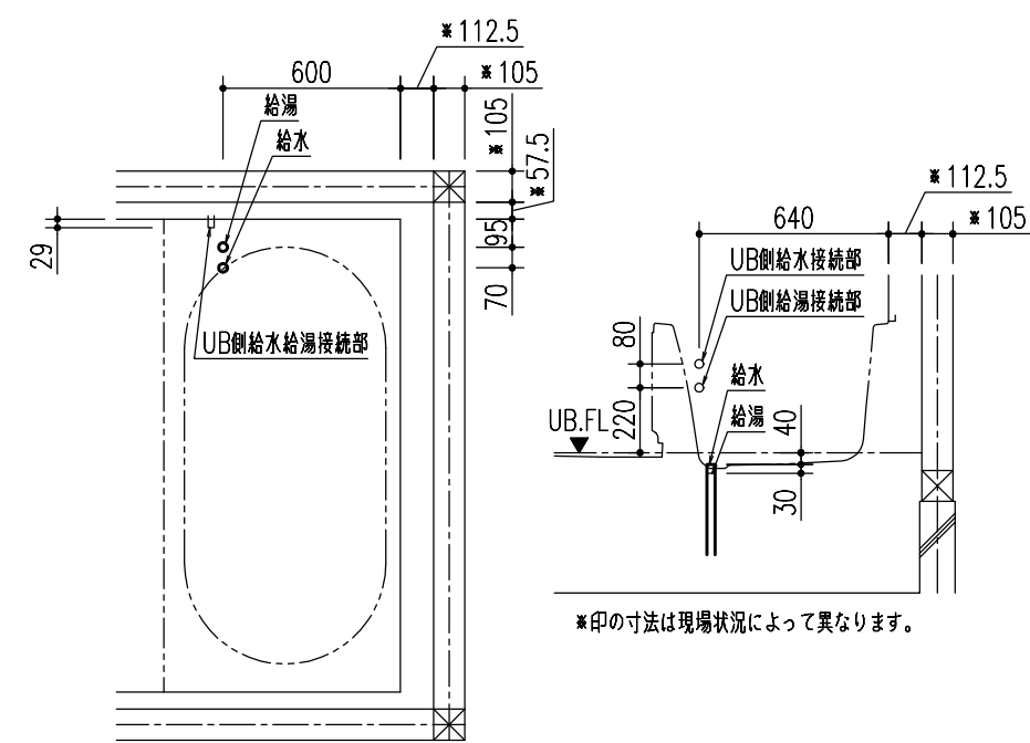
給水給湯配管立上げ位置 点検口止め
