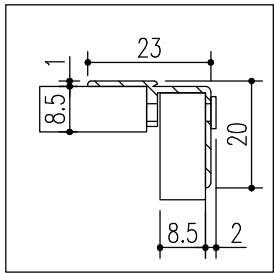
A矢視（上端接合部）
