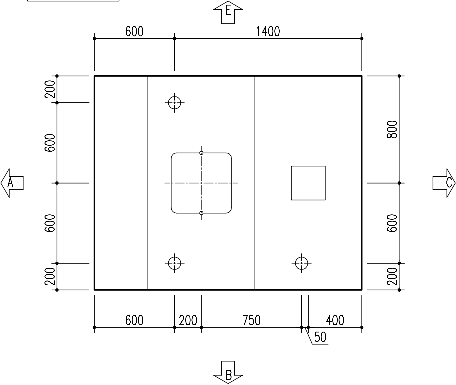
天井見上げ図
