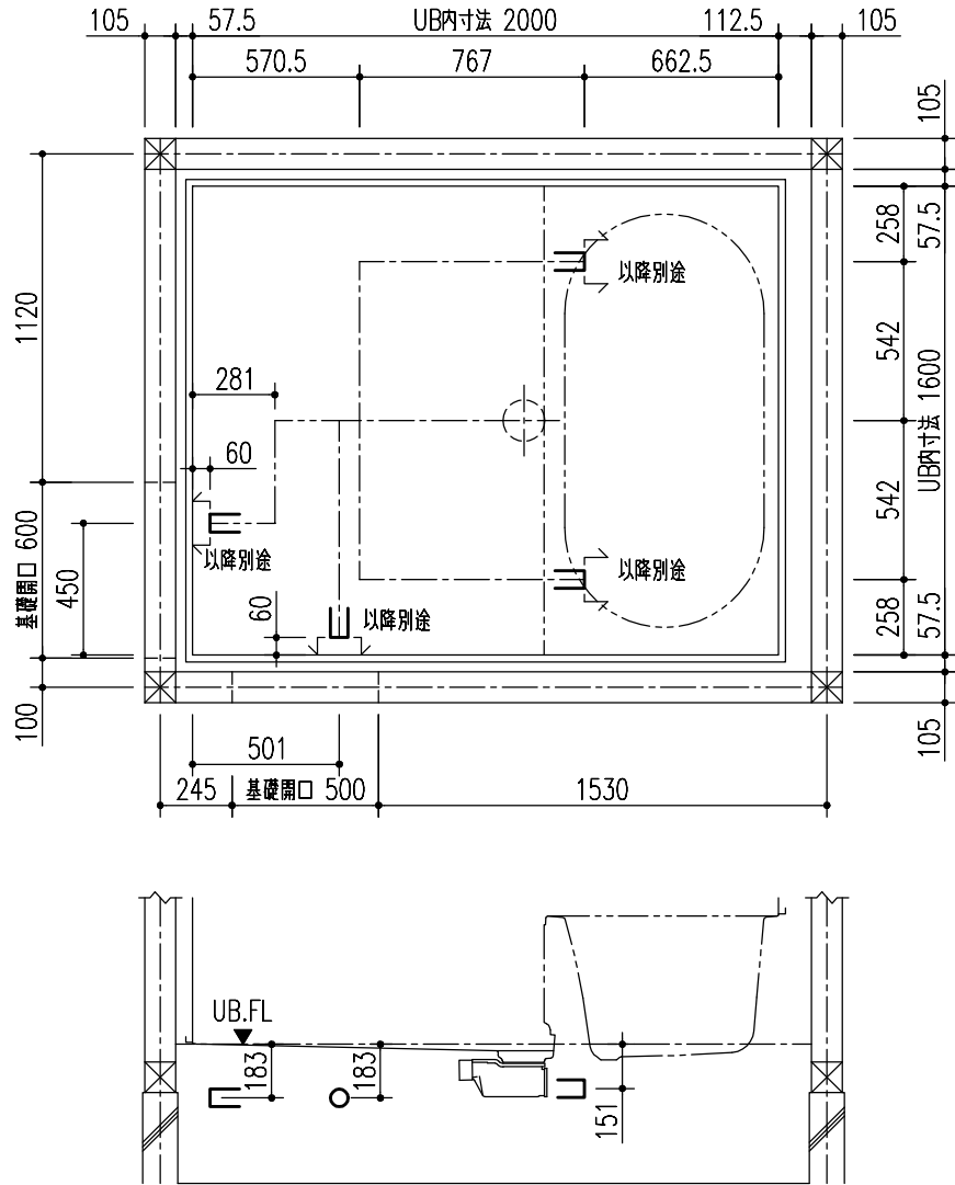
標準持出し位置
